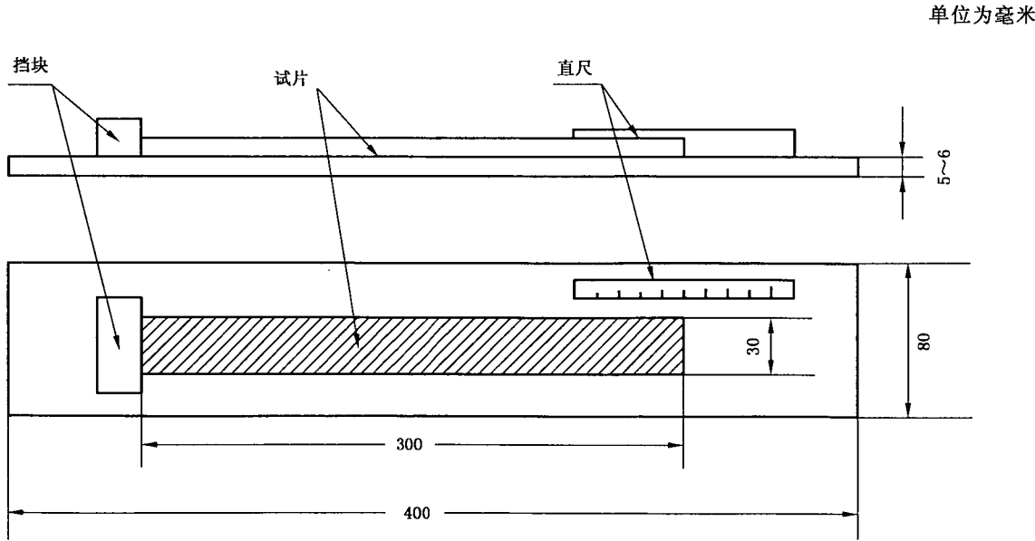
图 C.1 测量方法示意图
