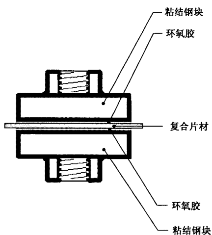
图 E.1 复合强度试件示意图
