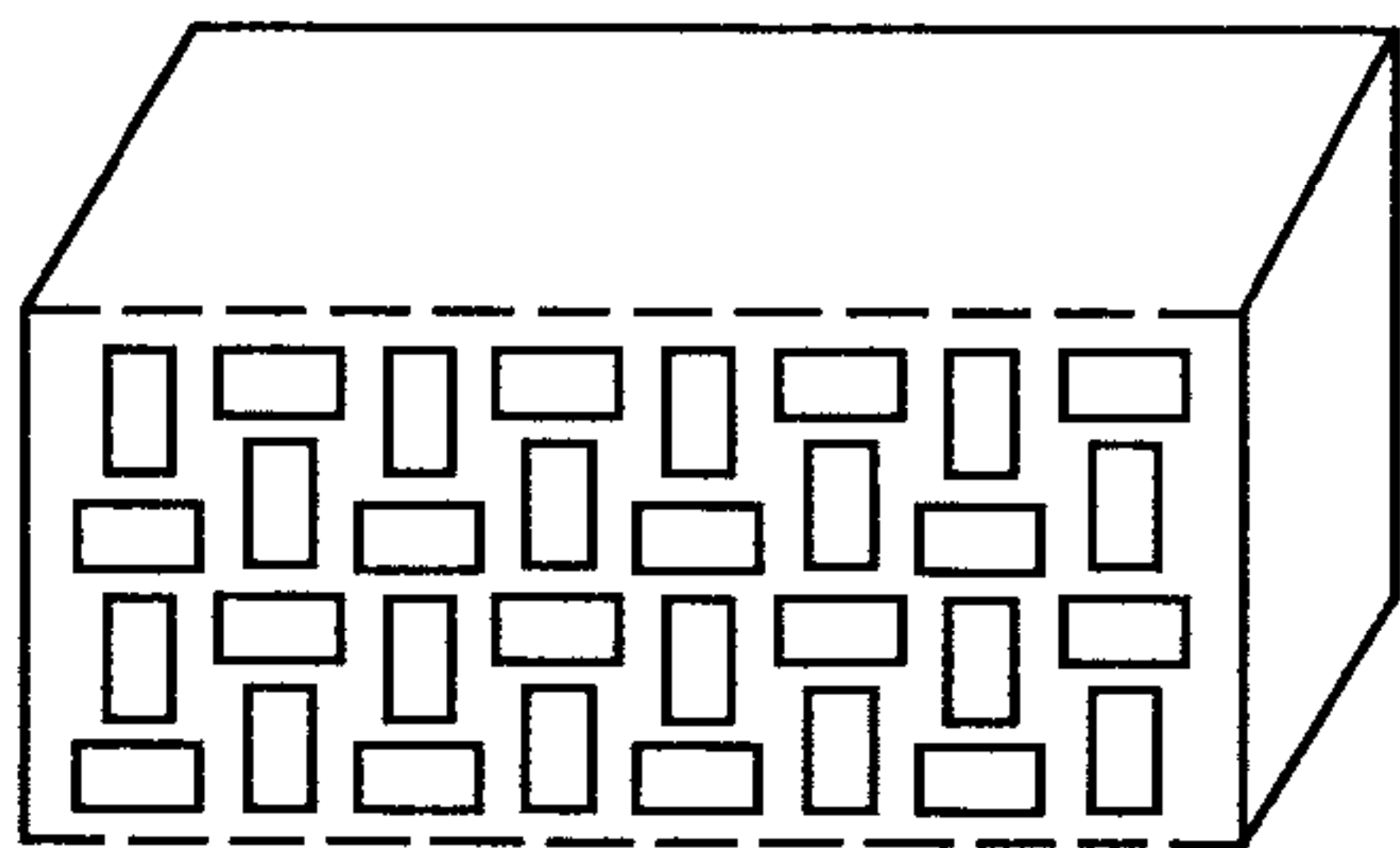
图 B.2 砖孔洞排列示意图
