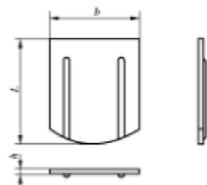
图 4 双筒瓦类
