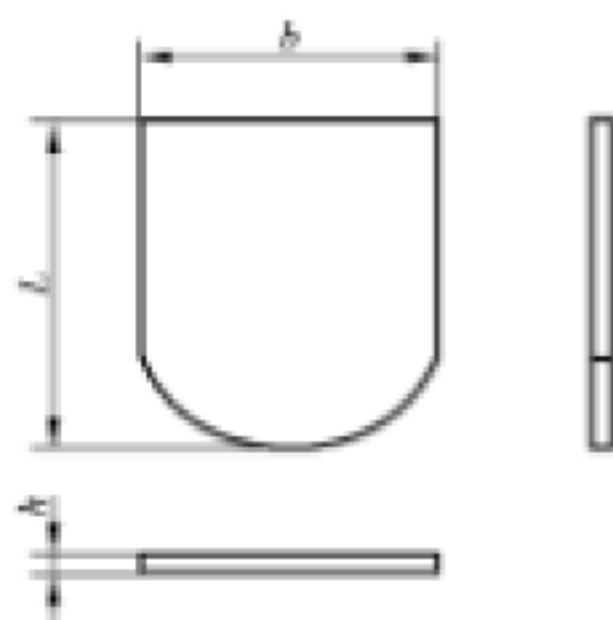
图 3 三曲瓦类
