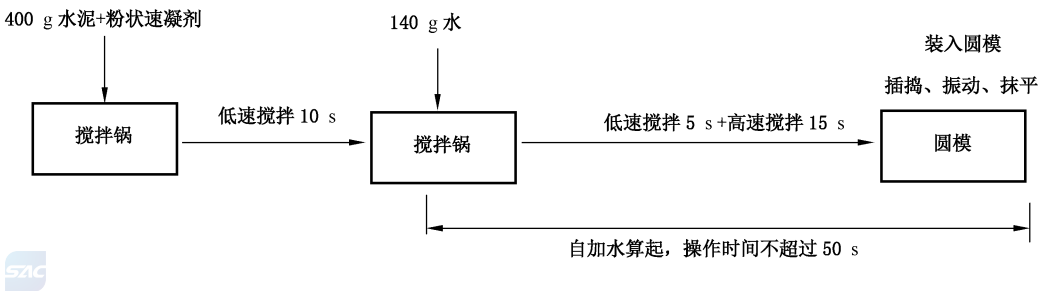
图 D.1 掺粉状速凝剂净浆凝结时间试验操作流程
